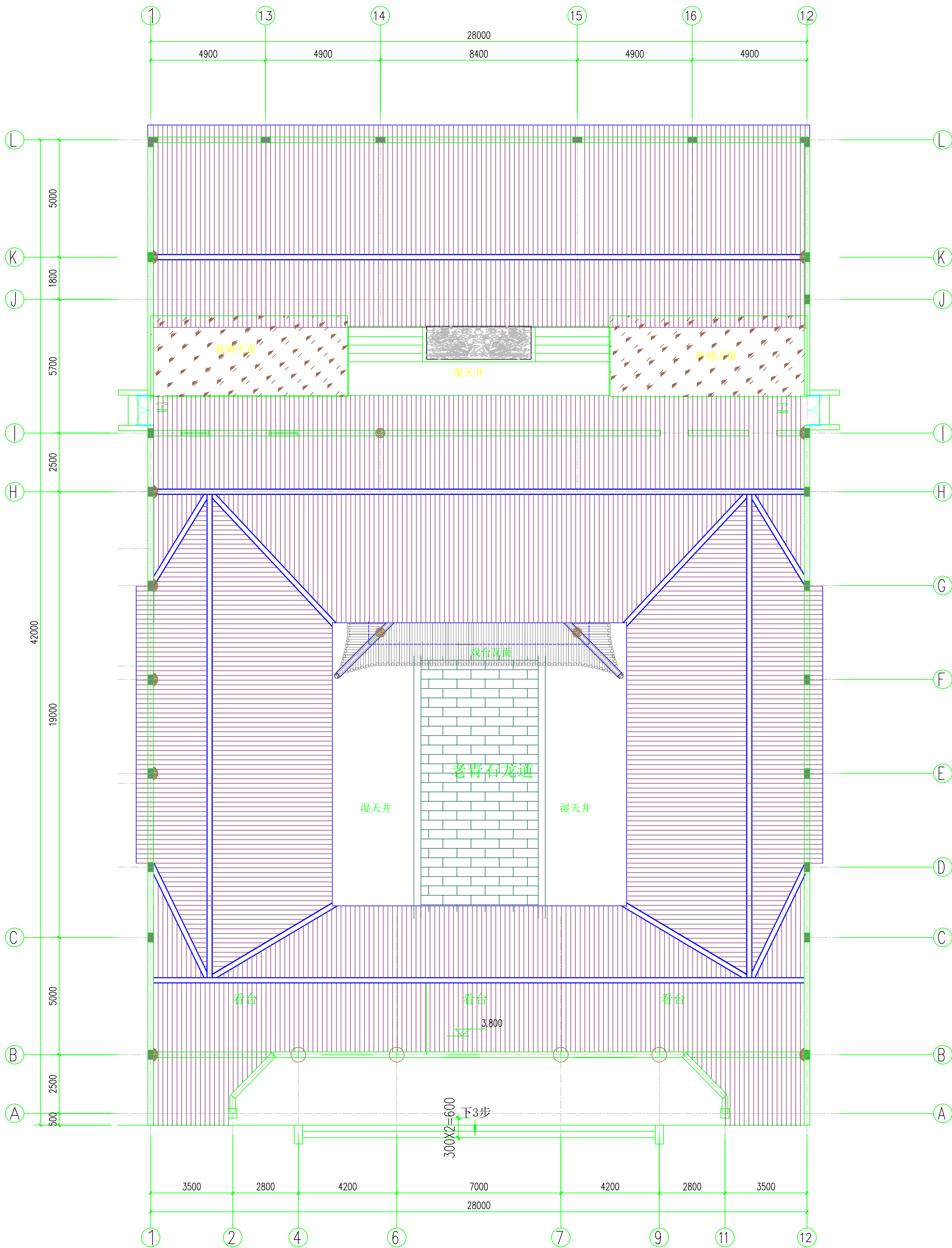
屋面俯视图 1:100
